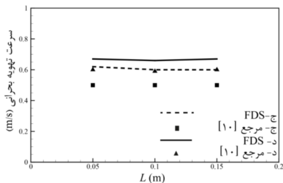
شکل ۶ مقایسه نتایج حاصل از شبیه‌سازی عددی با نتایج آزمایشگاهی تسای در حالت آرایش سه ردیف از خودروها
