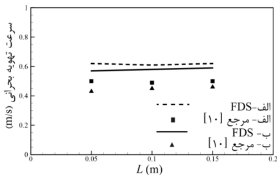
شکل ۷ ارزیابی نتایج حاصل از شبیه‌سازی عددی با نتایج آزمایشگاهی تسای در حالت آرایش دو ردیف از خودروها
