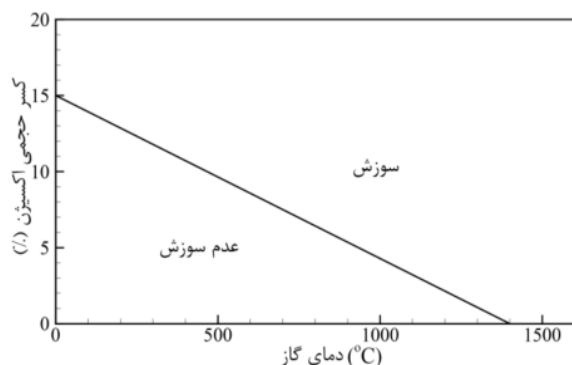
شکل ۲ نمودار غلظت حجمی اکسیژن بر حسب دما برای شعله‌وری و عدم شعله‌وری [۱۷]
