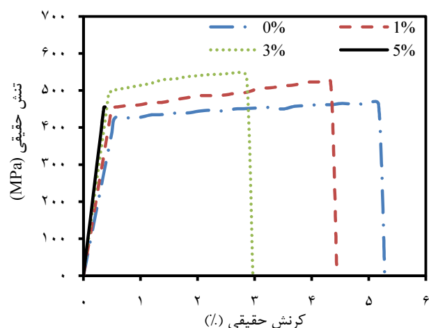
شکل ۷ آزمون فشار نانوکامپوزیت با زمینه آلومینیوم آلیاژی
