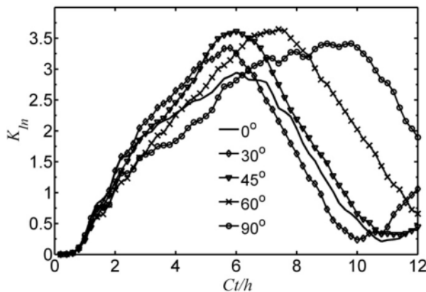
شکل ۷ مقدار ضریب شدت تنش بی بعد K_{In} در زمان‌های مختلف با زوایای ناهمسانگردی مختلف در ماده ارتوتروپیک
