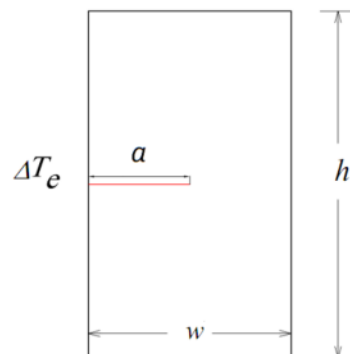
شکل ۳ صفحه ایزوتروپیک دارای ترک لبه‌ای تحت بارگذاری حرارتی
