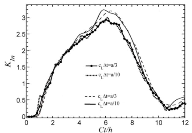
شکل ۹ مقدار ضریب شدت تنش بی بعد K_{In} در زمان‌های مختلف با زاویه ناهمسانگردی صفر درجه در ماده ارتوتروپیک
