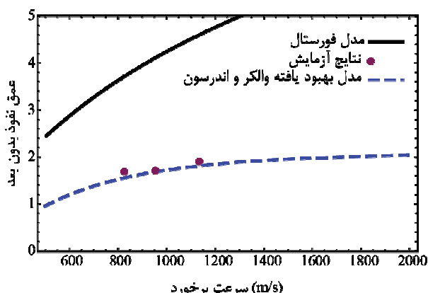
شکل ۱۲ تغییرات عمق نفوذ نهایی بر حسب سرعت برخورد- مقایسه مدل تحلیلی، نتایج آزمایش‌های تجربی هدف N-SF-0.3 و مدل فورستال
