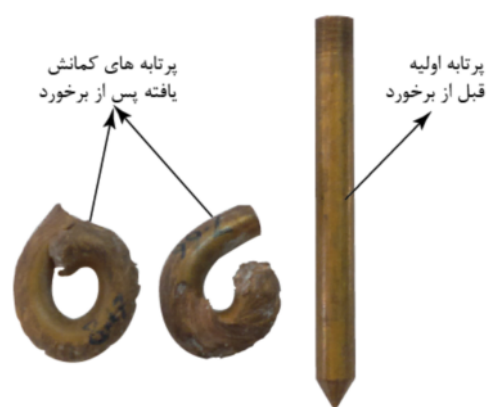
شکل ۸ پرتابه میله بلند فرسایشی پس از کمانش
