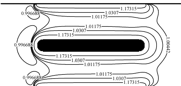
ج- خطوط هم تراز غلظت یون مثبت
