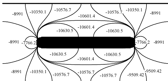
شکل ۹ خطوط هم تراز شدت میدان الکتریکی خارجی در مجراهای موازی
