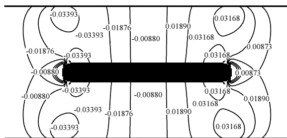
الف- خطوط هم تراز فشار
