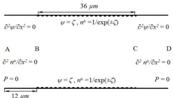
شکل ۱ هندسه و شرایط مرزی جریان الکترواسموتیک
