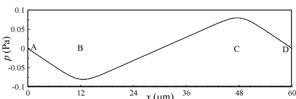
شکل ۵ تغییرات فشار نسبی در خط مرکزی مجرا
