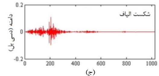
شکل ۸ سه سیگنال نمونه از مکانیزم‌های شکست؛ ترک خوردن ماتریس، لغزش الیاف و شکست الیاف
