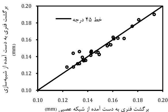
شکل ۱۵ مقایسه بین نتایج شبیه‌سازی و مقادیر پیش‌بینی شده توسط شبکه عصبی برای مقدار برگشت فنری
