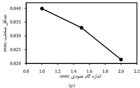
شکل ۸ تأثیر الف- ضریب اصطکاک، ب- اندازه قطر ابزار و ج- اندازه گام عمودی بر حداقل ضخامت ورق
