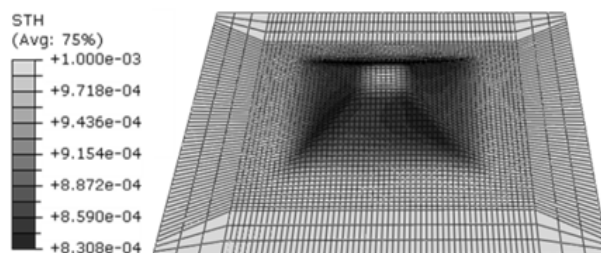
شکل ۷ توزیع ضخامت در مدل شبیه‌سازی شده با ضریب اصطکاک 0.05 ، قطر ابزار 15\text{ mm} میلی‌متر و اندازه گام عمودی 1/5\text{ mm} میلی‌متر
