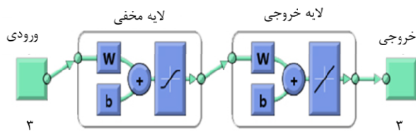
شکل ۱۲ شبکه عصبی طراحی شده برای مدل‌سازی نتایج شبیه‌سازی
