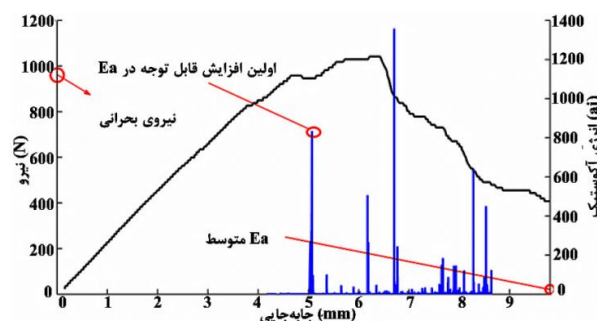
شکل ۶ به دست آوردن نیروی بحرانی برای قطعه A1 با استفاده از تکنیک توزیع انرژی
