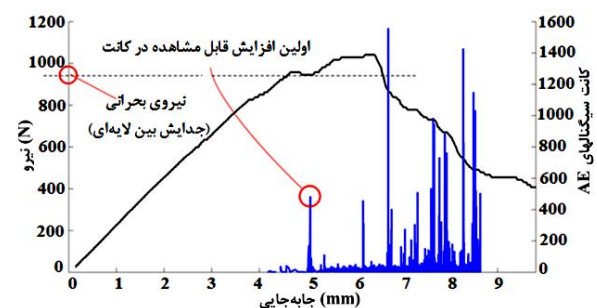
شکل ۸ به دست آوردن نیروی بحرانی برای قطعه A1 با استفاده از تکنیک توزیع کانت
