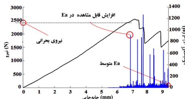
شکل ۷ به دست آوردن نیروی بحرانی برای قطعه A2 با استفاده از تکنیک توزیع انرژی
