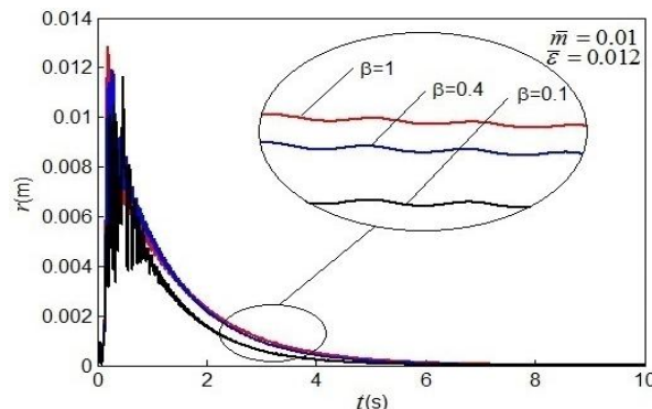
شکل ۱۷ پاسخ زمانی دامنه سیستم برای ضریب میرایی‌های مختلف
