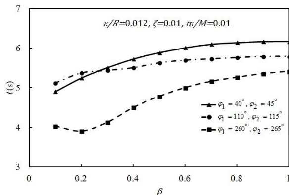
شکل ۱۶ زمان لازم برای میرا شدن دامنه حرکت بر حسب ضریب میرایی
