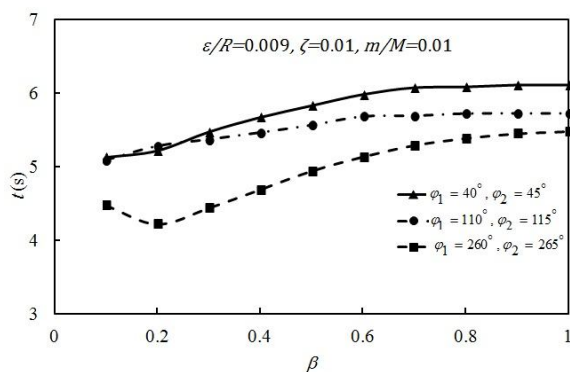
شکل ۹ زمان لازم برای میرا شدن دامنه حرکت بر حسب ضریب میرایی
