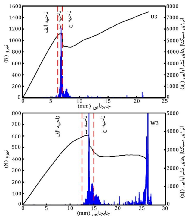
شکل 11 نمودار نیرو- انرژی سیگنال‌های نشرآوایی - جابجایی برای نمونه U3 و W3
