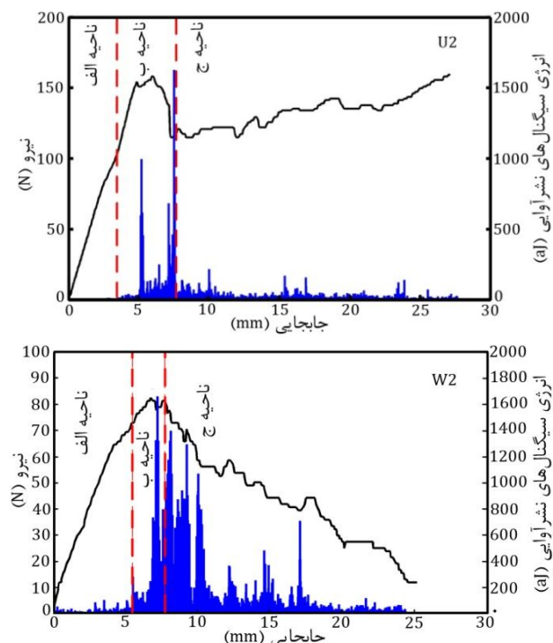
شکل 10 نمودار نیرو- انرژی سیگنال‌های نشرآوایی - جابجایی برای نمونه U2 و W2
