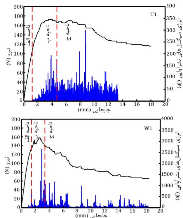
شکل 9 نمودار نیرو- انرژی سیگنال‌های نشرآوایی - جابجایی برای نمونه U1 و W1
