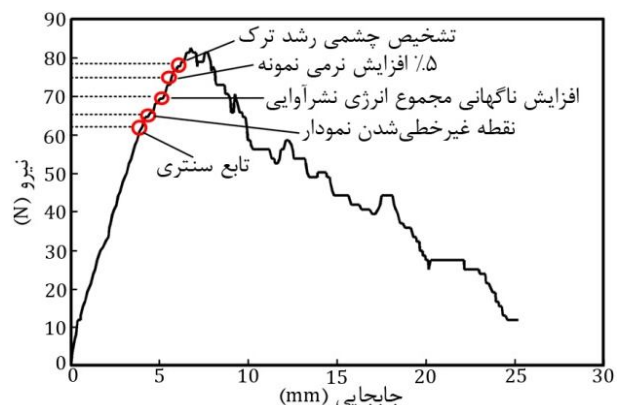
شکل 22 مقادیر بار بحرانی بدست آمده برای نمونه W2، با روش‌های مکانیکی، نشر آوایی و آکوستومکانیکی
