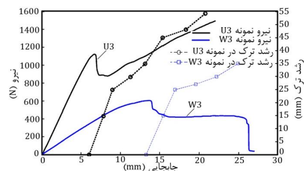
شکل 5 منحنی نیرو-رشد ترک-جابجایی برای نمونه‌های U3 و W3
