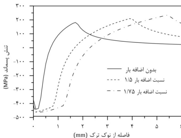
شکل 15 توزیع تنش پسماند فشاری نوک ترک
