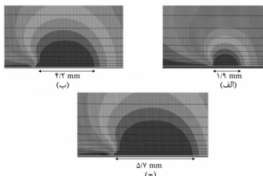
شکل 14 اندازه ناحیه پلاستیک نوک ترک در (الف) بارگذاری بدون اضافه بار، (ب) اعمال اضافه بار با نسبت 1/5 و (ج) اضافه بار با نسبت 1/75
