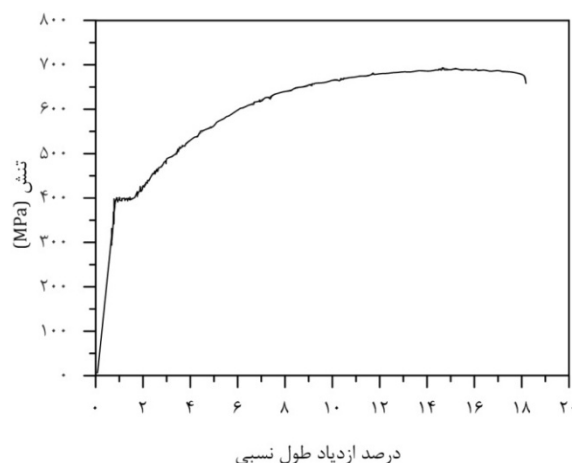
شکل 1 تست کشش نمونه استاندارد E8 فولاد AISI 4140
