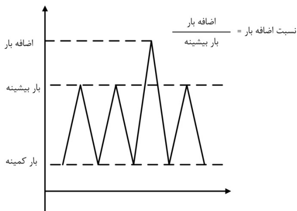
شکل 4 نحوه اعمال اضافه بار
