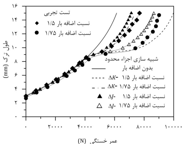
شکل 18 پیش‌بینی عمر خستگی مدل‌های اجزاء محدود
