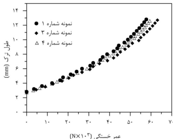
شکل 9 نتایج تجربی آزمون رشد ترک نمونه استاندارد CT از فولاد AISI 4140
