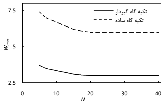
شکل ۱۸ جابه‌جایی مرکز صفحه به‌ازای مقادیر مختلف تعداد گره‌های به‌کار رفته برای آنالیز حساسیت مش
