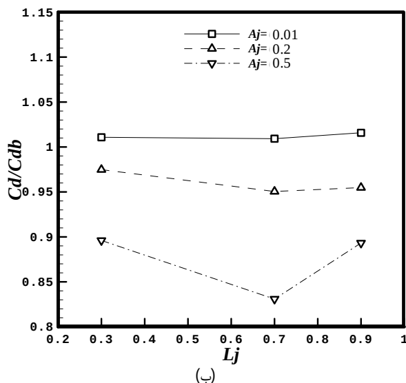
شکل 7 نتایج عددی ضریب برآ و پسا در عدد رینولدز 2000 و زاویه حمله 10 درجه و زاویه دمش 90 درجه: (الف) ضریب برآ، (ب) ضریب پسا
