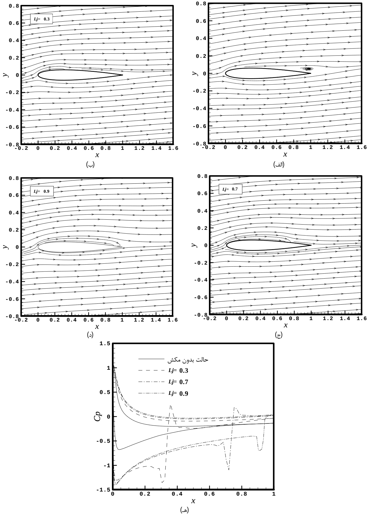
شکل 15 اثر مکش بر خطوط جریان و توزیع فشار در عدد رینولدز 2000 و زاویه حمله 5 درجه: الف) حالت بدون مکش، ب) L_j = 0/3 ، ج) L_j = 0/7 ، د) L_j = 0/9 ، ه) توزیع فشار روی سطح
