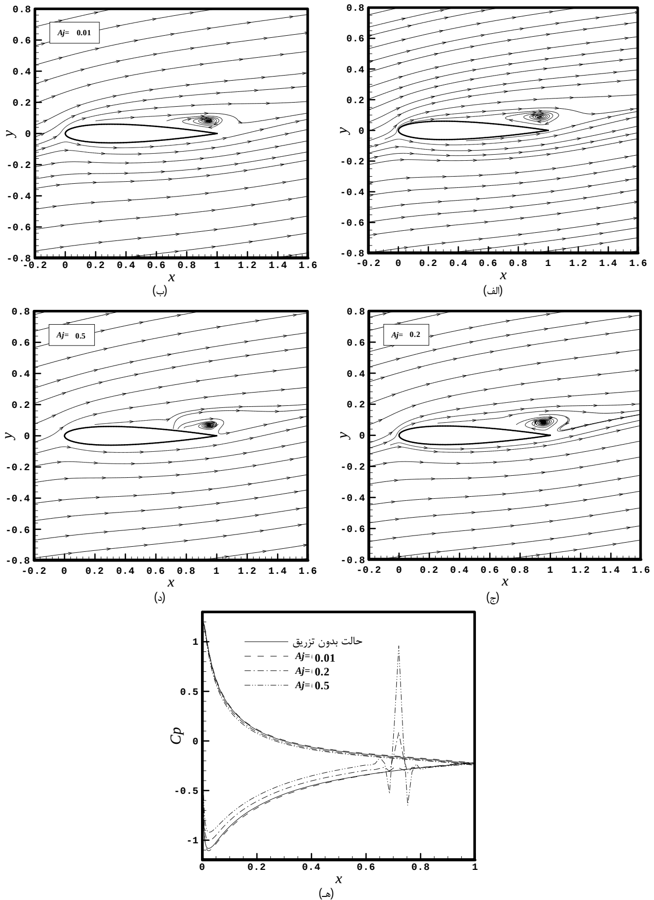
شکل 10 اثر دمش بر خطوط جریان و توزیع فشار در عدد رینولدز 500 و زاویه حمله 10 درجه: الف) حالت بدون تزریق، ب) A_j = 0/01 ، ج) A_j = 0/2 ، د) A_j = 0/5 ، ه) توزیع فشار روی سطح
