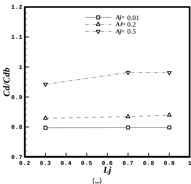
شکل 13 نتایج عددی ضریب برآ و پسا در عدد رینولدز 2000، زاویه حمله 5 درجه و زاویه مکش 90 درجه: الف) ضریب برآ، ب) ضریب پسا
