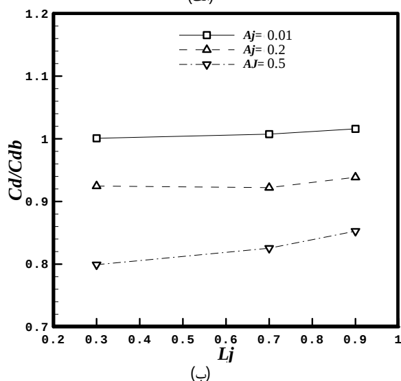
شکل 8 نتایج عددی ضریب برآ و پسا در عدد رینولدز 2000، زاویه حمله 10 درجه و زاویه دمش 30 درجه: (الف) ضریب برآ، (ب) ضریب پسا
