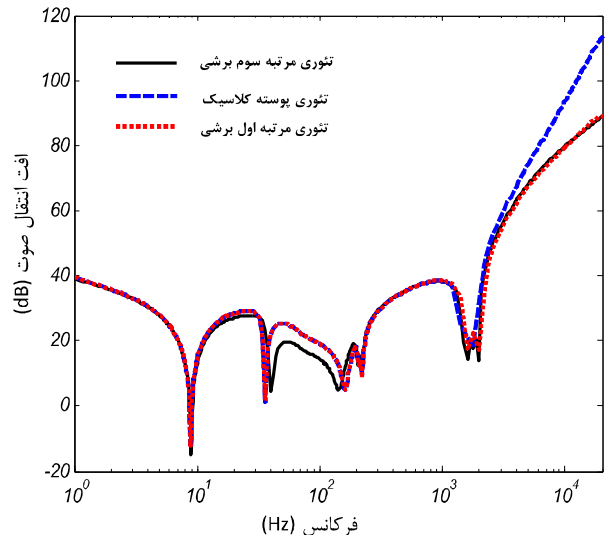
شکل 7 مقایسه نتایج TSDT با نتایج CST و FSDT برای R/h=100
