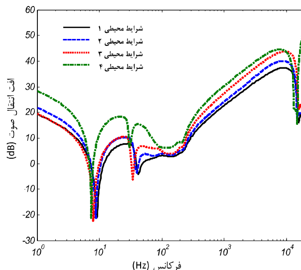
شکل 12 بررسی شرایط محیطی بر افت انتقال صوت پوسته استوانه‌ای
