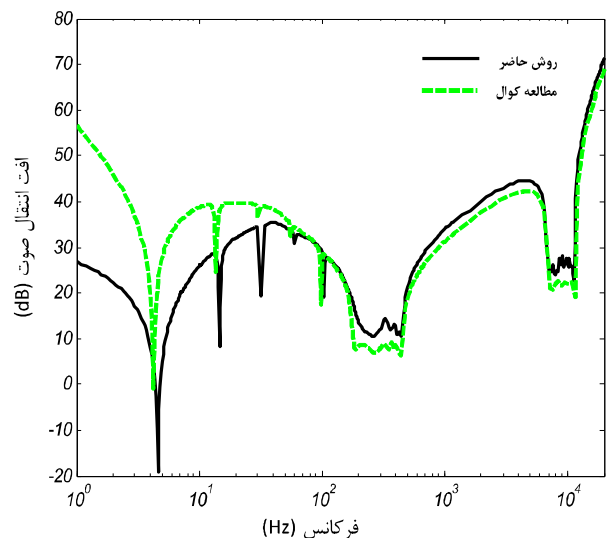
شکل 5 مقایسه افت انتقال صوت بین روش حاضر و نتایج کوال [5]
