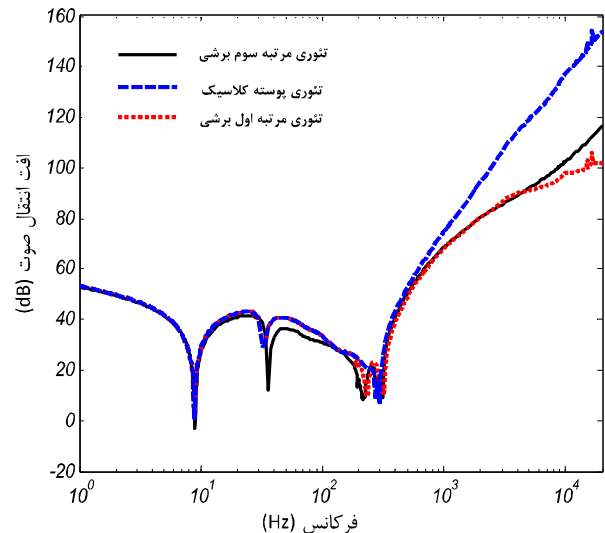
شکل 8 مقایسه نتایج TSDT با نتایج CST و FSDT برای R/h=20
