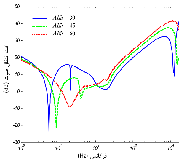
شکل 11 بررسی تغییر زاویه برخورد بر افت انتقال صوت پوسته استوانه‌ای
