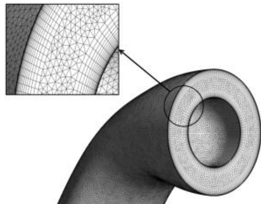
شکل ۱۵ شبکه بی‌سازمان با شبکه بندی لایه مرزی
