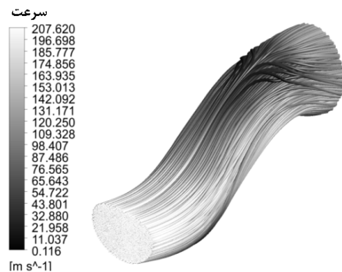
شکل ۲۵ خطوط جریان در مجرا سه بعدی با مقاطع لوبیایی
