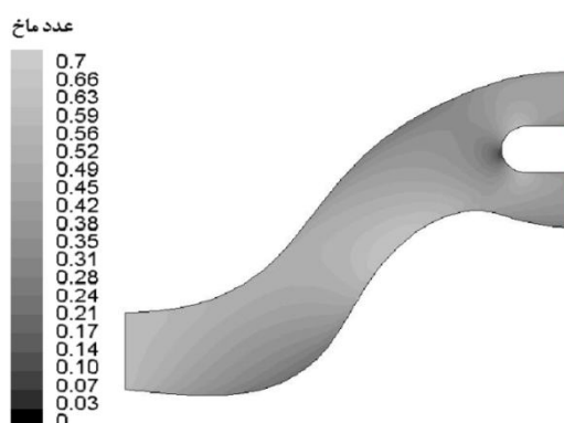
شکل ۱۱ کانتر عدد ماخ برای هندسه دوبعدی طراحی شده
