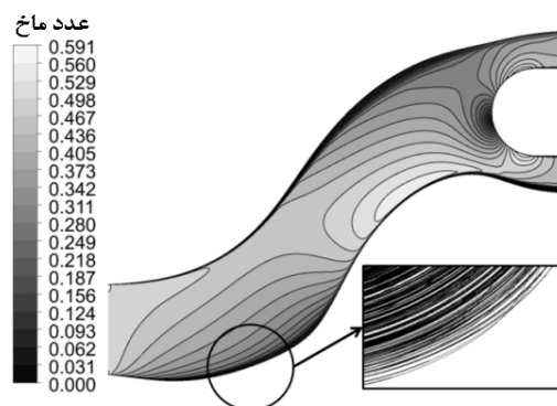
شکل ۲۶ کانتور بردارهای سرعت روی مقطع تقارن مجرای سه بعدی اصلاح شده با مقاطع لوبیایی
