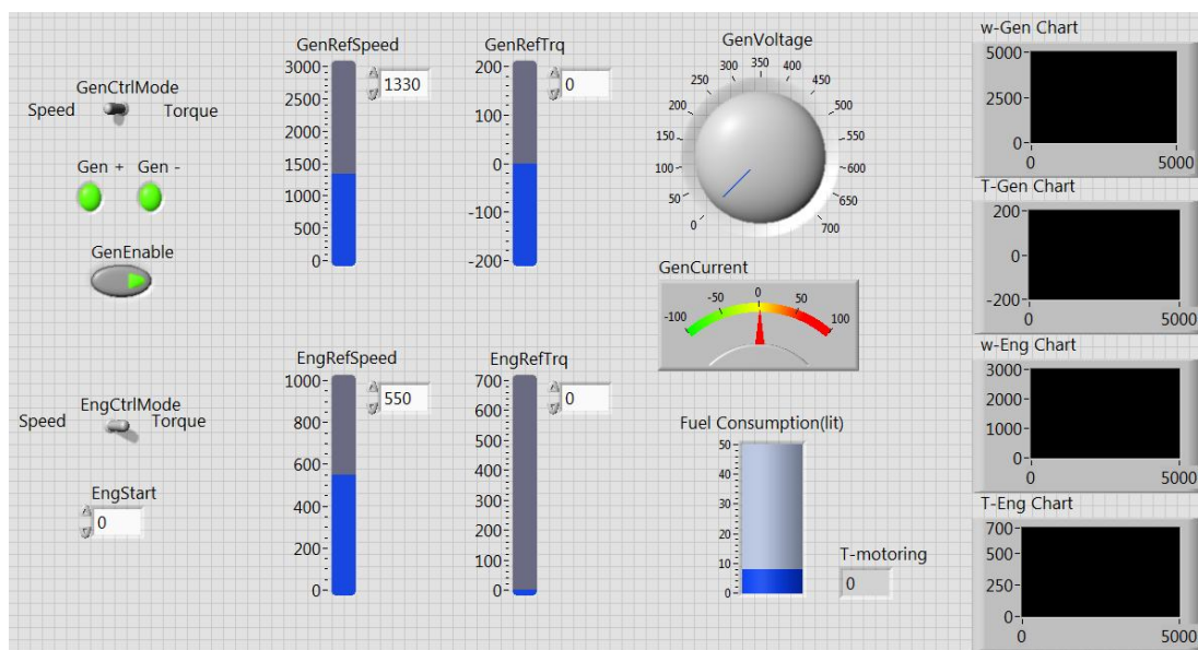
شکل ۸ پانل جلویی شبیه‌ساز مجموعه تولید توان
