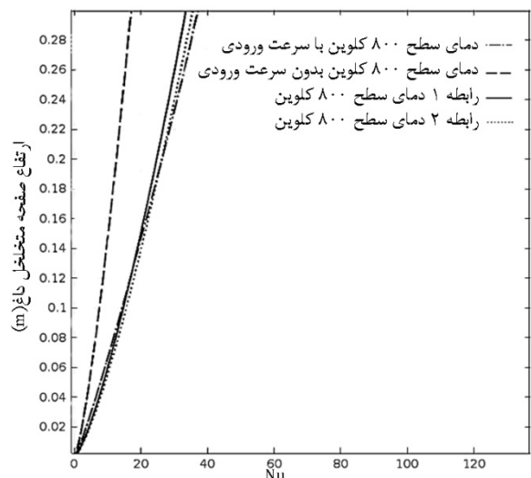
شکل ۱۰ مقایسه عدد ناسلت برای دمای سطح برابر با ۸۰۰ کلوین از مدل‌سازی و دو رابطه تجربی
