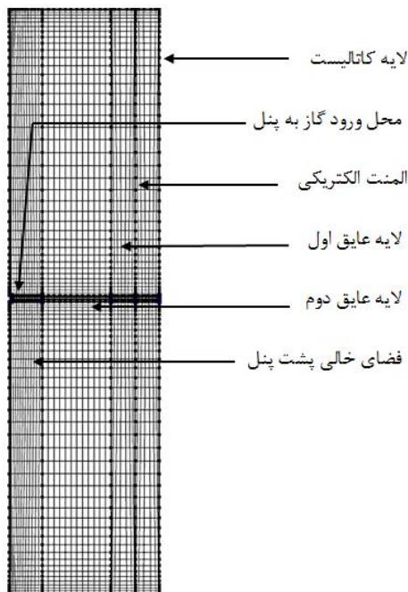
شکل ۲ هندسه و شبکه‌بندی مشعل تشعشعی کاتالیستی به صورت دوبعدی
