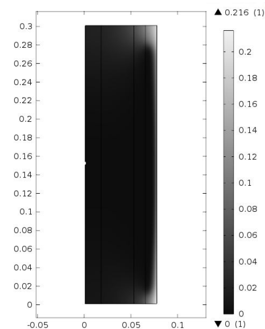
شکل ۱۲ توزیع کسر جرمی اکسیژن در مشعل با دبی گاز ۴/۹۳ lit/min
