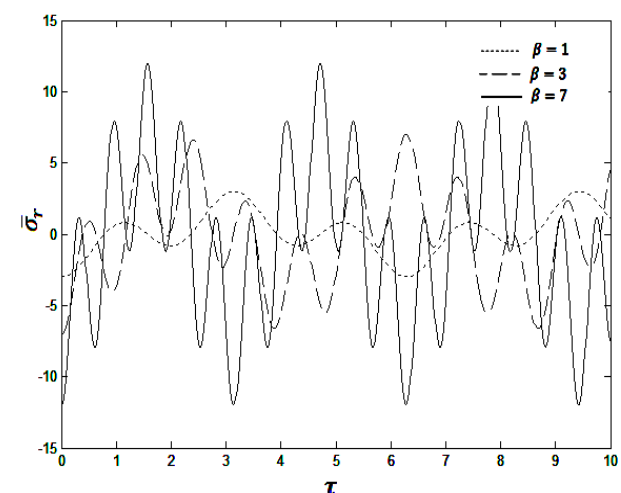
شکل ۱۰ تغییرات زمانی تنش شعاعی نسبت به تغییرات \beta در نقطه وسط استوانه برای استوانه‌ای با شرایط شکل ۴
