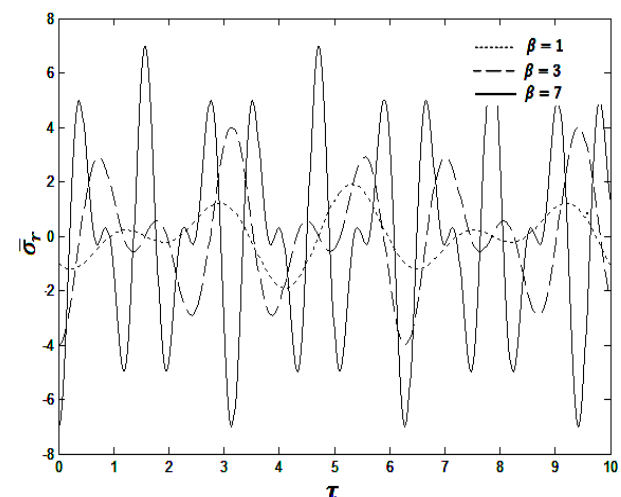
شکل ۹ تغییرات زمانی تنش شعاعی نسبت به تغییرات \beta در محل اتصال لایه‌های
