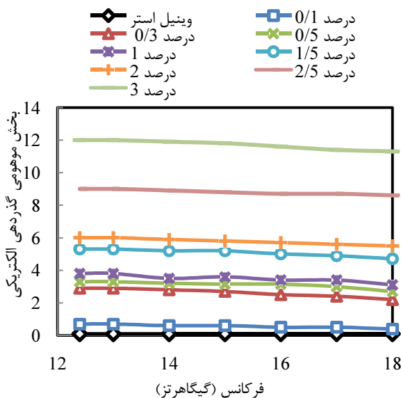
شکل ۹ بخش موهومی گذردهی الکتریکی نانوکامپوزیت در باند فرکانسی Ku برای ۵۰ دقیقه التراسونیک از ۰/۱ تا ۳ درصد کسر وزنی نانولوله کربن چنددیواره و رزین خالص
