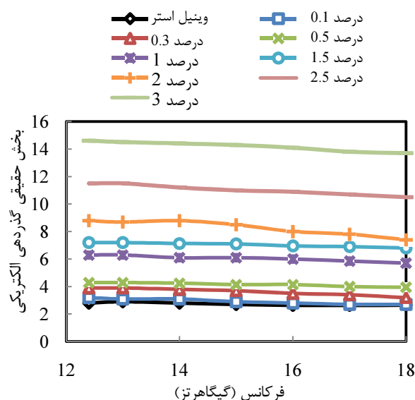
شکل ۸ بخش حقیقی گذردهی الکتریکی نانوکامپوزیت در باند فرکانسی Ku برای ۵۰ دقیقه التراسونیک از ۰/۱ تا ۳ درصد کسر وزنی نانولوله کربن چنددیواره و رزین خالص
