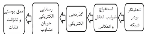
شکل ۶ شمای کلی فرایند استخراج خواص الکتریکی و الکترومغناطیسی
