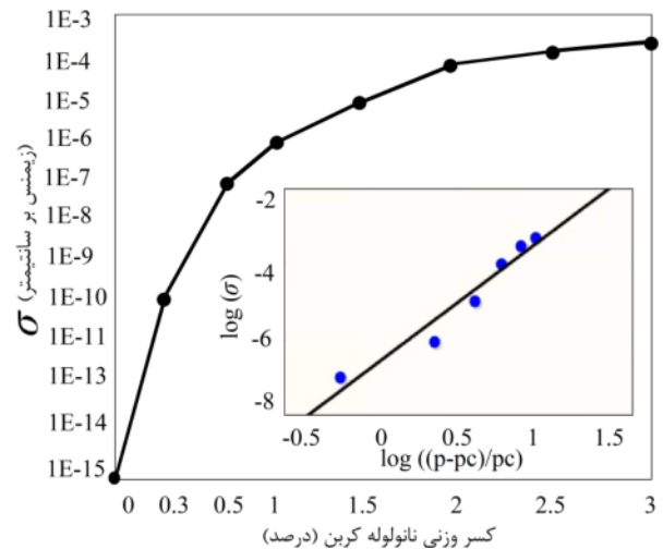
شکل ۷ میزان رسانایی الکتریکی جریان مستقیم نانوکامپوزیت نانولوله کربنی/وینیل استر بر حسب کسر وزنی نانولوله کربنی
