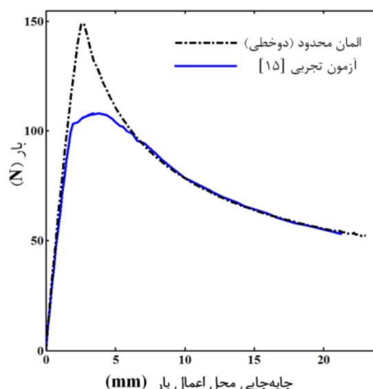
شکل ۱۵ پیش‌بینی منحنی بار-جابجایی با استفاده از مدل ناحیه چسبناک دوخطی
