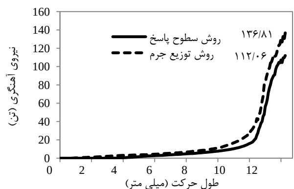
شکل ۹ منحنی نیرو-جابجایی در دو حالت آهنگری با پیش‌فرم سنتی و پیش‌فرم بهینه‌سازی شده به روش سطوح پاسخ
