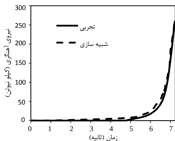
شکل ۱۸ نمودار نیرو-زمان مربوط به نتایج شبیه‌سازی و آزمایش‌های تجربی
