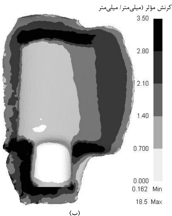
شکل ۱۰ مقایسه توزیع کرنش در دو حالت طراحی، الف- مدل بهینه شده توسط روش سطوح پاسخ، ب- روش سنتی توزیع جرم
