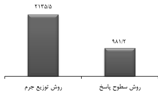
شکل ۸ مقایسه حجم پلیسه (میلی‌متر مکعب) در دو حالت طراحی با روش سنتی توزیع جرم و مدل بهینه شده توسط روش سطوح پاسخ
