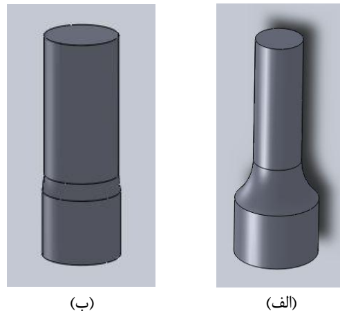
شکل ۳ مدل پیش‌فرم‌های الف- حداقل، ب- حداکثر
