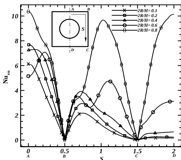
شکل ۸ توزیع ناسلت محلی روی دیواره‌های محفظه بسته مربعی در حضور استوانه دایروی با نسبت‌های 2R/H مختلف در رایلی 10^5
