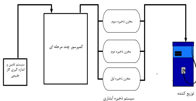
شکل ۱ شماتیک یک ایستگاه سوخت CNG
