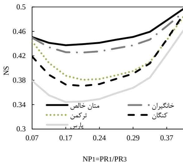
شکل ۱۰ تأثیر عدد NP_1 بر NS
