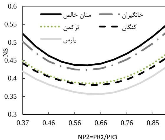
شکل ۱۱ تأثیر عدد NP_2 بر NS
