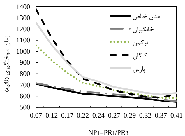
شکل ۸ تأثیر عدد NP_1 بر زمان سوخت‌گیری
