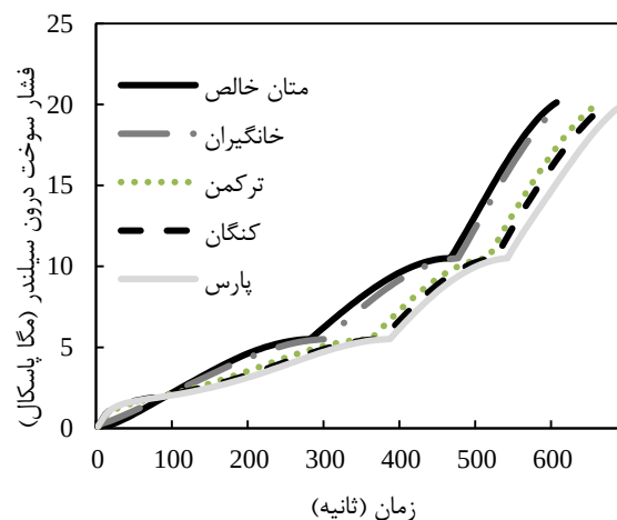
شکل ۴ تغییرات فشار سوخت درون مخزن CNG بر حسب ترکیب‌های مختلف گاز طبیعی
