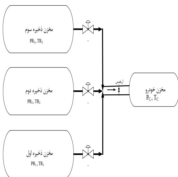
شکل ۲ شماتیک مخازن ذخیره آبشاری و مخزن خودرو
