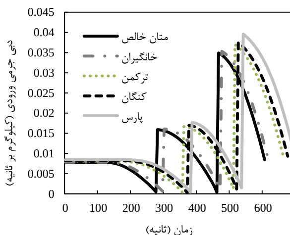
شکل ۵ تغییرات دبی جرمی سوخت درون مخزن CNG بر حسب ترکیبات مختلف گاز طبیعی
