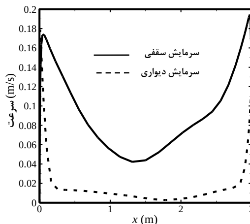
شکل ۷ توزیع سرعت مطلق هوا در راستای افقی وسط اتاق مدل‌های A و B؛ دمای سطح سرد 17^{\circ}\text{C} و دمای طرح خارج 38^{\circ}\text{C}
