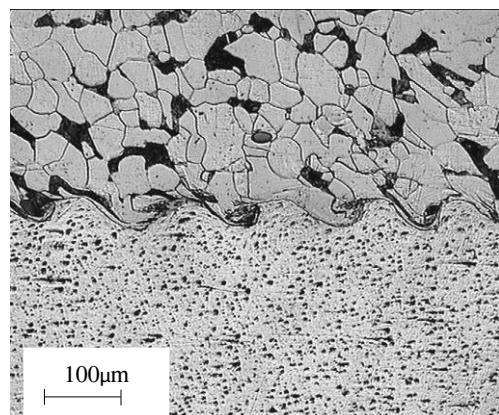
شکل ۱۵ مرز مشترک جوش دو فلز (به ترتیب از بالا ۱۵/۵ و ۱۸ گرم «آماتول ۹۵-۵»، بزرگنمایی ۲۰۰ برابر و ۱۰۰ برابر [۷])
