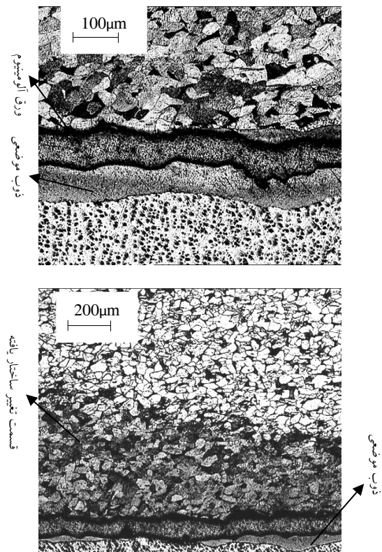
شکل ۸ مرز مشترک جوش دو فلز (۲۳ گرم TNT) لایه بالا: فولاد St-۳۷، لایه پایین: فسفر- برنز، بزرگنمایی به ترتیب از بالا ۱۰۰X و ۵۰X [۷]
