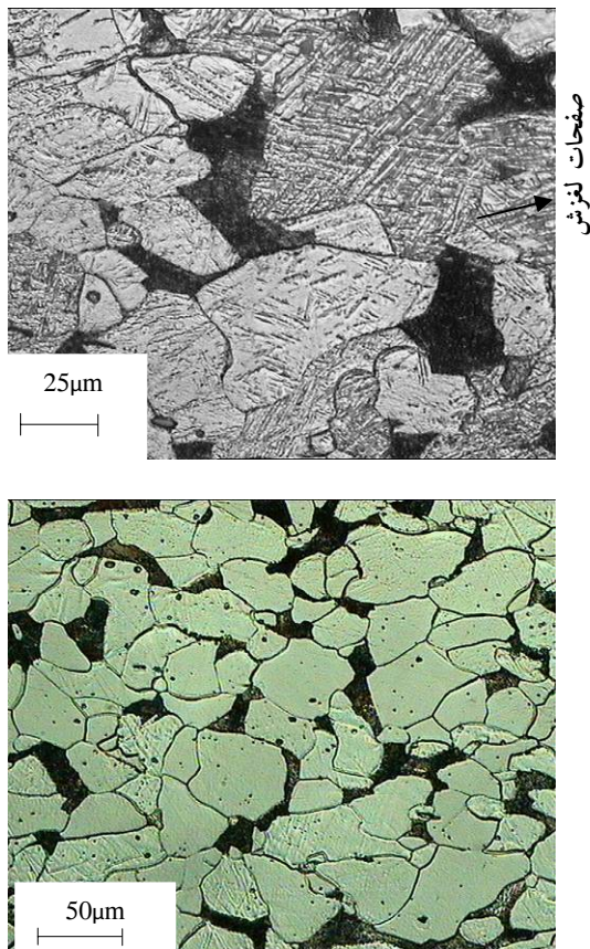
شکل ۹ تصویر متالوگرافی از قسمت فولادی، نزدیک و دور از فصل مشترک، بزرگنمایی به ترتیب از بالا ۴۰۰X و ۲۰۰X [۷]
