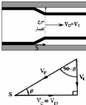
شکل ۲ دیاگرام سینماتیکی پارامترهای اصلی برخورد [۳]
