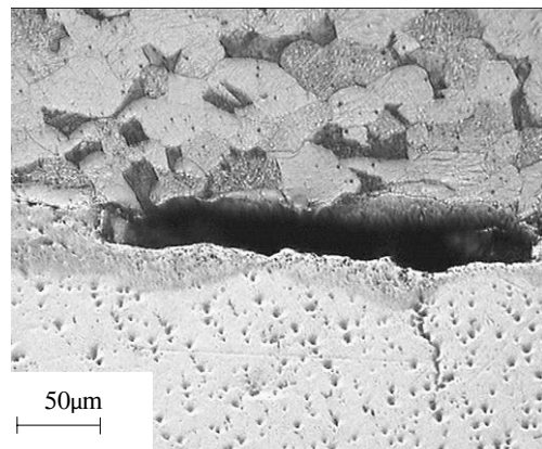
شکل ۱۱ مرز مشترک جوش دو فلز (۱۵/۵ گرم TNT)، بزرگنمایی به ترتیب بالا برابر ۱۰۰ و ۲۰۰ برابر [۷]
