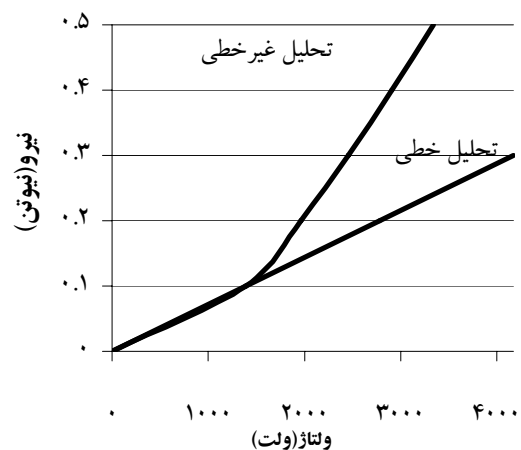
شکل ۷ مقایسه ولتاژ خطی و غیرخطی تیر
