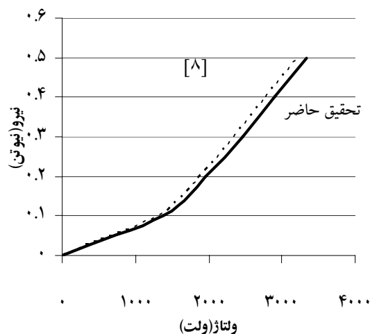
شکل ۵ مقایسه ولتاژ غیر خطی تحقیق حاضر با [۸]
