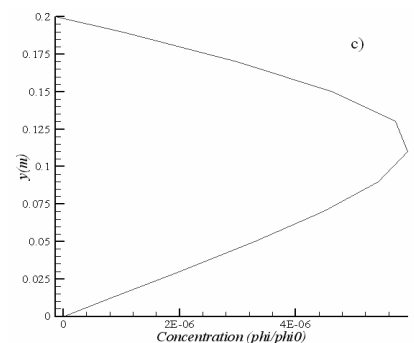
شکل ۶ تأثیر عدد Re بر انتقال خاصیت در جریان پشت پله
