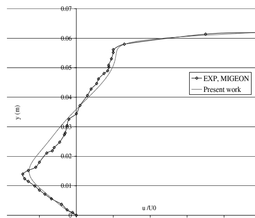
شکل ۴ مقایسه مقادیر آزمایشگاهی و حل سرعت افقی در محور تقارن عمودی حفره
