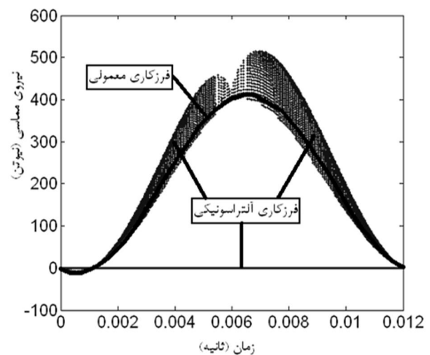
شکل 4 نیروی برشی مماسی در فرزکاری معمولی و آلتراسونیک با پارامترهای N=2500 rpm، K_t=5000 N/mm 2 ، a_a=0.4 mm، a_{tz}=0.2 mm/tooth، Z=4 ، D=10 mm، f=23 kHz و a=20 \mu m
