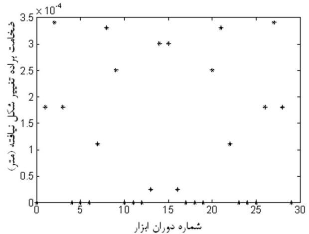
شکل 2 ضخامت براده تغییر شکل نیافته در موقعیت زاویه‌ای \theta=30^\circ در 30 دور گردش متوالی ابزار با شرایط f=21732 Hz و a=5 \mu m، N=500 rpm
