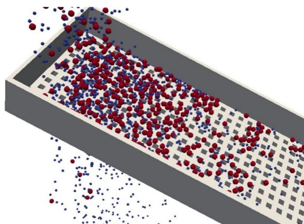
شکل 6 لحظه ای از حرکت ذرات روی توری سرنده طی یک شبیه سازی
