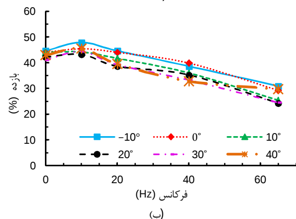
شکل 7 نمودارهای وابستگی بازده به فرکانس برای زوایای مختلف ارتعاشی (مختلف به ازای الف) شیب \beta = 5^\circ و (ب) شیب \beta = 10^\circ
