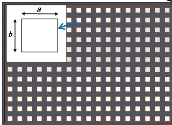
شکل 2 تعریف پارامترهای شیب، راستای تحریک ارتعاش خطی و روزنه‌های توری سرنده
