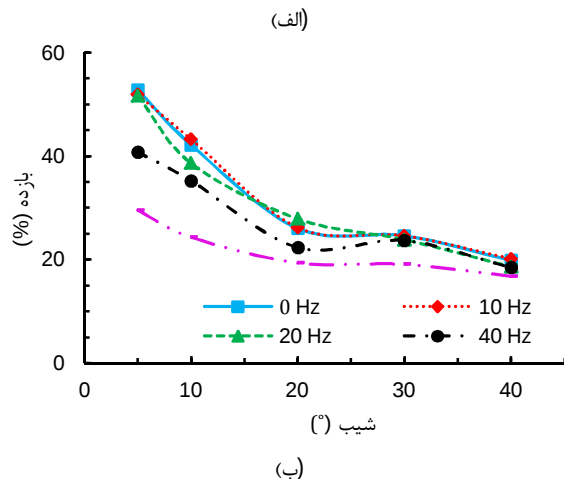
شکل 8 نمودارهای تغییرات بازده بر حسب زاویه شیب سرد و فرکانس‌های مختلف (به ازای الف) زاویه ارتعاش \alpha = -10^\circ و (ب) زاویه ارتعاش \alpha = 20^\circ
