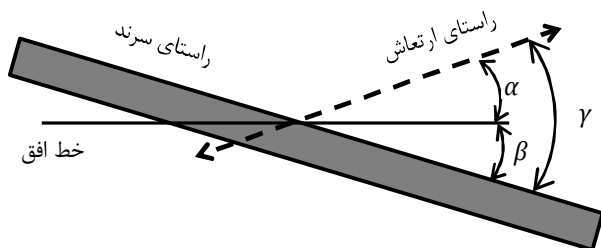
شکل 1 نمونه‌های حرکت ذرات با اندازه‌های بزرگ‌تر و کوچک‌تر از روزنه توری
