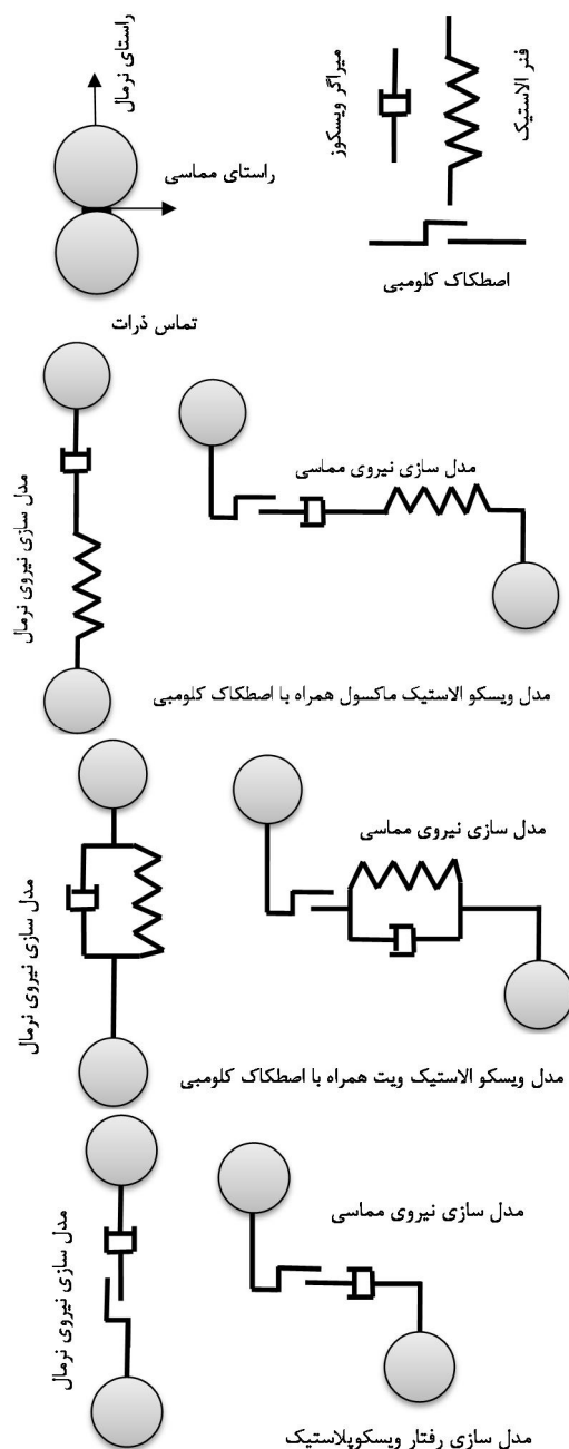
شکل 5 مدل‌سازی برخورد غیر الاستیک ذرات در بیان نیروهای نرمال و مماسی
