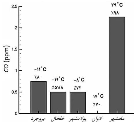
شکل 12 میزان نشر CO برای دبی سوخت 3/6 l/min در شرایط محیطی مختلف
