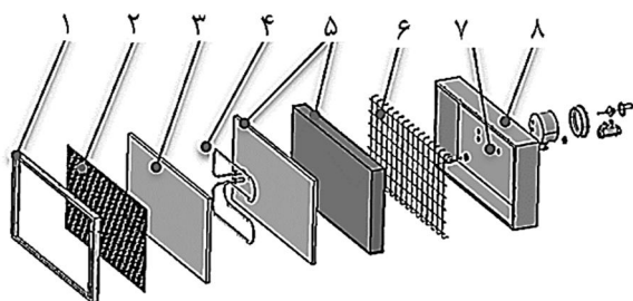
شکل 1 شماتیک پنل تشعشعی کاتالیستی. (1) قاب نگهدارنده، (2) توری، (3) لایه کاتالیستی، (4) المنت الکتریکی، (5) لایه عایق، (6) محفظه آرامش، (7) ورودی گاز، (8) بدنه پنل [3].
