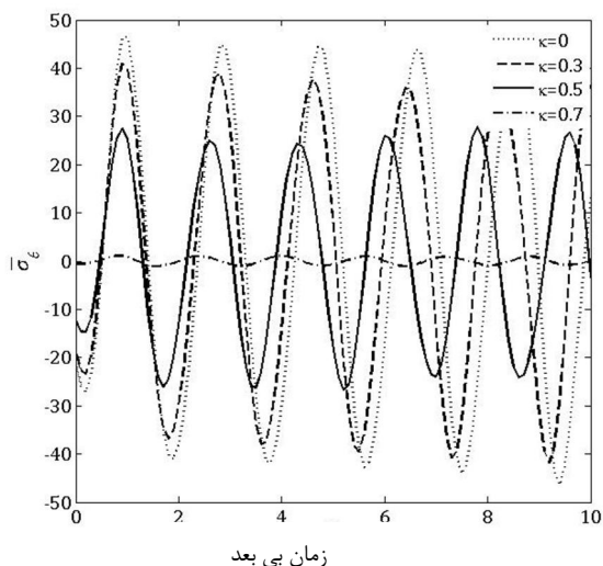
شکل 4 تغییرات زمانی تنش محیطی در صفحه داخلی
