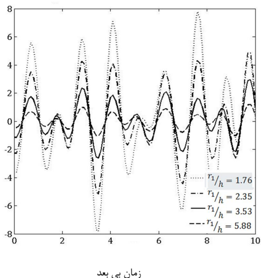
شکل 3 تغییرات زمانی تنش شعاعی در نقطه میانی در راستای شعاع
