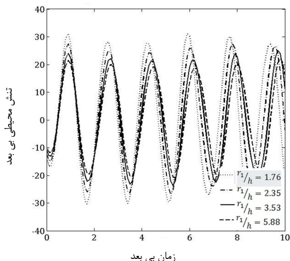
شکل 7 تغییرات زمانی تنش محیطی در سطح داخلی
