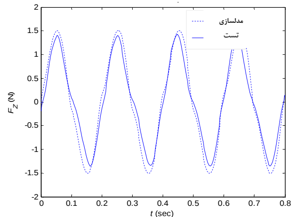
شکل 5 مقایسه نیروی جلوبرنده در مدل و آزمون
