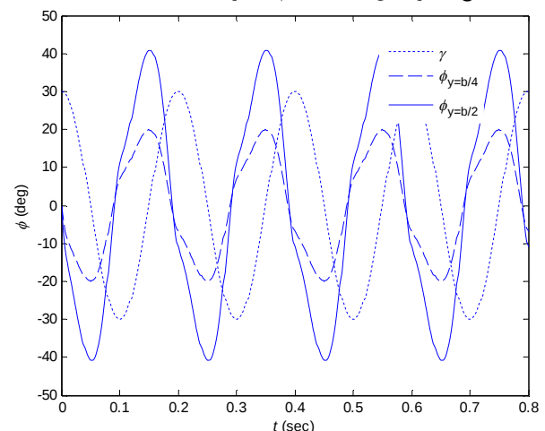
شکل 6 منحنی تغییرات پیچش برای میانه و نوک بال
