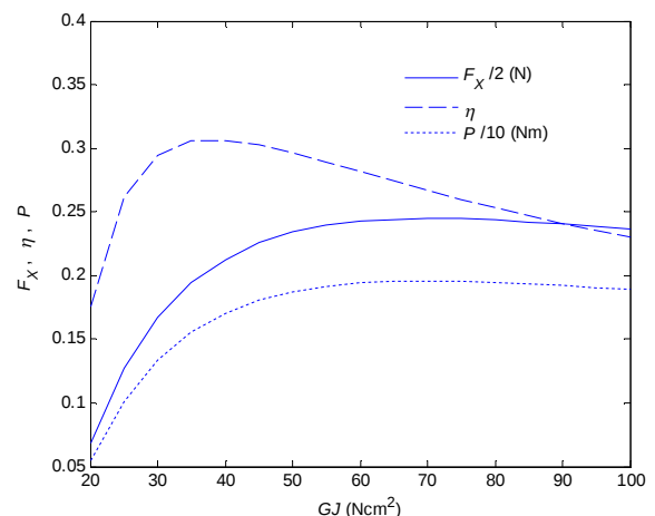
شکل 11 تغییر مشخصه پیشران بر حسب سختی پیچشی
