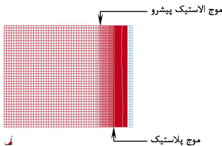
شکل 10 (الف) تشکیل موج شوک در ابتدای راه
