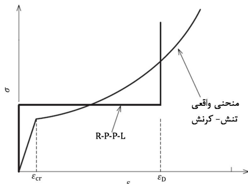
شکل 3 منحنی تنش - کرنش اسمی و مدل R-P-P-L [6]
