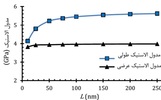
شکل 10 نمودار تغییرات مدول طولی و عرضی بر حسب طول نانولوله کربن به ازای کسر حجمی 1% نانولوله و نسبت b/D_0 = 1.75
