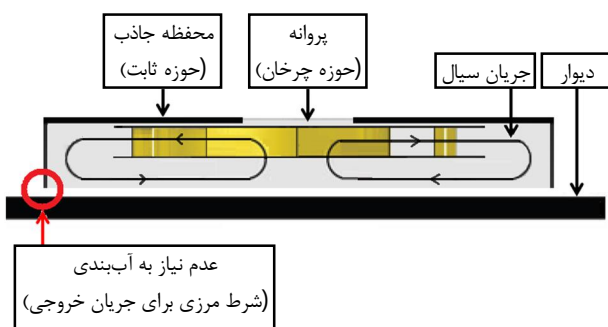
شکل 10 شکل شماتیک جاذب گردابه‌ای
