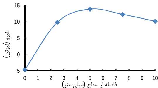
شکل 14 نیروی جاذبه تولیدی جاذب بر حسب فاصله از سطح در سرعت 12250 دور در دقیقه
