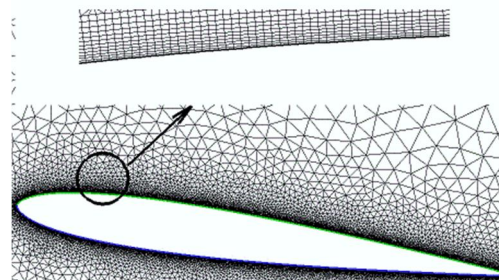
شکل 2 شبکه محاسباتی حول ایرفویل با اعمال لایه مرزی به دیواره
