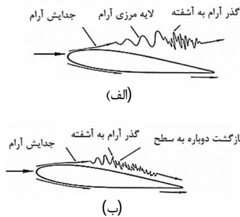
شکل 1- جریان حول ایرفویل با عدد رینولدز پایین [8] (الف) جدایش کامل و بدون بازگشت (ب) جدایش با بازگشت به سطح و تشکیل حباب جدایش
