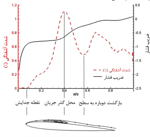
شکل 11 توزیع فشار و شدت آشفتگی جریان و محل تشکیل حباب جدایش تحت اثر سطح در زاویه حمله 5 درجه
