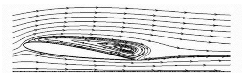
شکل 15 خطوط جریان در جریان تحت پدیده اثر سطح در زاویه حمله 8 درجه
