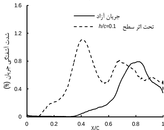
شکل 7 توزیع شدت آشفتگی سطح بالایی ایرفویل در جریان آزاد و تحت اثر سطح در زاویه حمله 5 درجه
