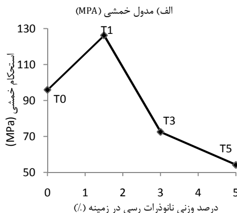
شکل ۵ تغییرات خواص خمشی نمونه‌های نانوکامپوزیتی
