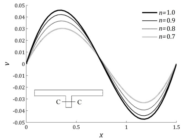
شکل ۱۰ سرعت عرضی سیال نیوتنی تعمیم یافته در y = \frac{3}{2} (امتداد خط C-C) و عدد رینولدز ۲۰ و به ازای توان نمایی n از 0.7 تا 1.0
