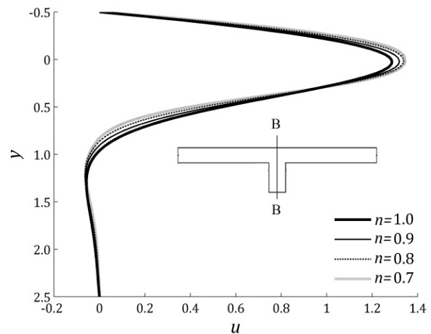
شکل ۹ پروفیل سرعت طولی سیال نیوتنی تعمیم یافته در x = \frac{1}{2} (امتداد خط B-B) و عدد رینولدز ۲۰ به ازای توان نمایی n از 0.7 تا 1.0
