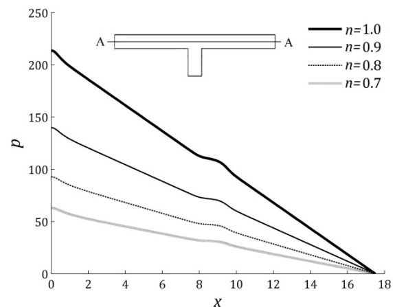
شکل ۹ توزیع فشار طولی سیال نیوتنی تعمیم‌یافته در y = 0 (امتداد خط A-A) به‌ازای رینولدز ۲۰ و توان نمایی n از ۱/۰ تا ۱/۰
