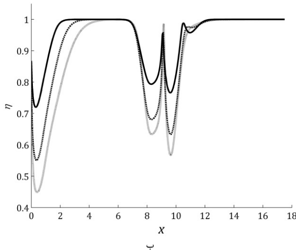
شکل ۷ توزیع الف) نرخ برش تعمیم یافته و ب) لزجت بدون بعد سیال نیوتنی تعمیم یافته در y = 0 (امتداد خط A-A) برای عدد رینولدز ۲۰ و به ازای مقادیر توان نمایی 0.7 تا 0.9
