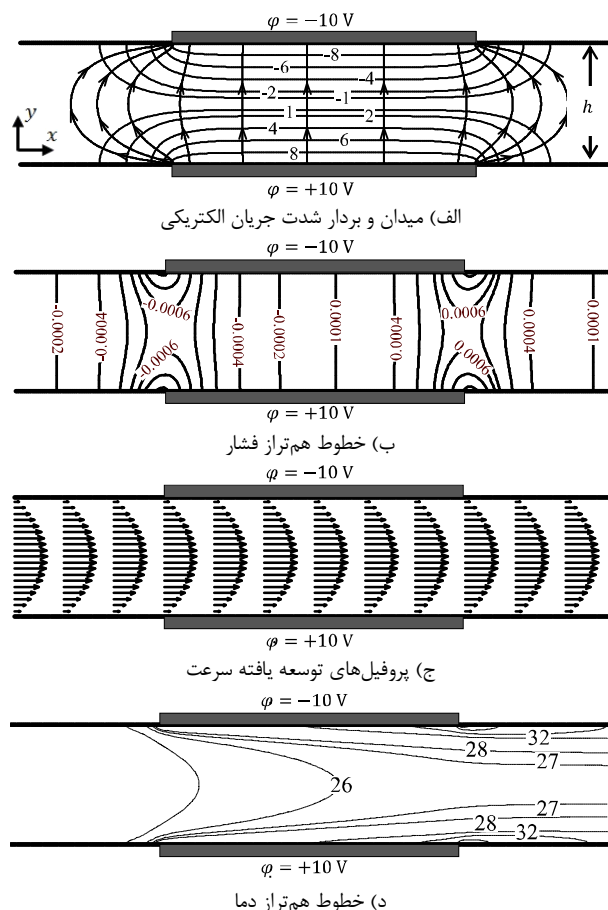
شکل ۸ نتایج عددی در z = b/2 ، (الف) خطوط میدان و بردار شدت جریان الکتریکی، (ب) میدان فشار، (ج) میدان سرعت، (د) میدان دما
