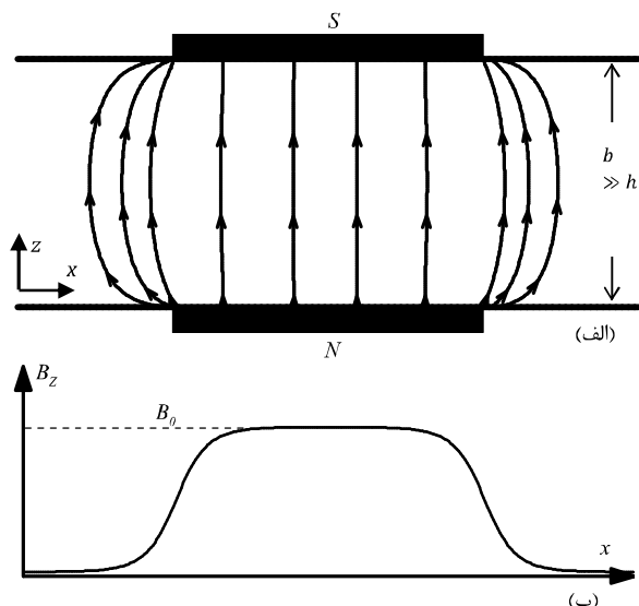
شکل ۷ نتایج عددی، (الف) خطوط میدان مغناطیسی در صفحه xz ، (ب) تغییرات B_z در راستای x در z = b/2
