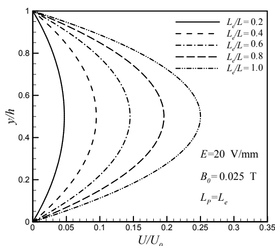
شکل ۱۰ توزیع سرعت به ازای تغییر طول میدان الکتریکی و مغناطیسی (خواص ثابت)
