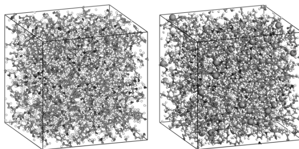
شکل ۲ ساختار مدل‌های EP00 بدون اتصالات عرضی و EP64 با اتصالات عرضی پلیمر اپوکسی با اتصالات عرضی ترکیب رزین اپوکسی و سخت‌گر
