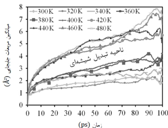
شکل ۳ نمودارهای MSD-زمان برای اپوکسی در دماهای مختلف با فواصل 20 K، تعیین‌کننده محدوده دمای تبدیل شیشه‌ای
