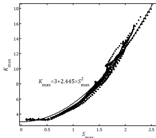
شکل ۱۴ نمودار تغییرات بیشینه کورتوسیس مولفه ناهمگن سرعت برحسب تغییرات بیشینه اسکینوس این مولفه (این نتیجه تطبیق خوبی با [۲۳] دارد.)
