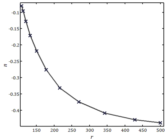
شکل ۸ نمودار تغییرات توان استهلاک انرژی جنبشی برحسب تغییرات ضریب طول انتگرالی، r
