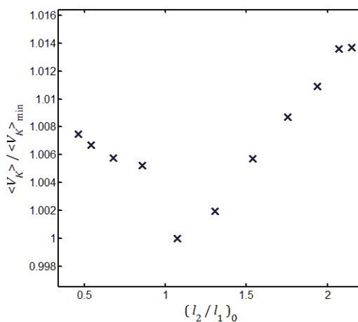
شکل ۲۰ نمودار تغییرات متوسط زمانی واریانس شعاع انحنای انرژی برحسب تغییرات نسبت طول انتگرالی اولیه (نقاط با اندازه نقطه کمینه، بی‌بعد شده‌اند).
