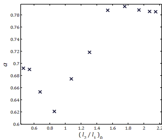
شکل ۱۸ تغییرات توان پخش آشفتگی برحسب تغییرات نسبت طول انتگرالی در لحظه اولیه
