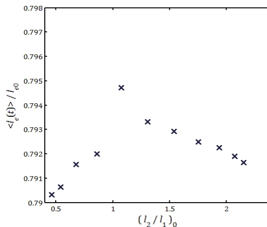
شکل ۱۹ تغییرات متوسط زمانی طول لایه اختلاط انرژی برحسب تغییر نسبت طول انتگرالی اولیه
