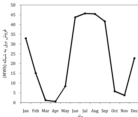
شکل ۱۰ برق فروخته شده به شبکه توسط سیستم تولید همزمان در ماه‌های مختلف
