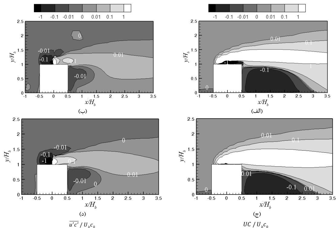
شکل ۸ کانتورهای شار جابه‌جایی بی‌بعد UC / U_b c_0 و شار بی‌بعد دیفیوژن آشفتگی \overline{u'c'} / U_b c_0 برای مدل‌های (الف) و (ب) اِرهارد و موسیوپولاس و (ج) و (د) k-\varepsilon استاندارد در صفحه z / H_b = 0
