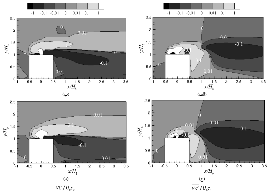
شکل ۹ کانتورهای شار جابه‌جایی بی‌بعد VC / U_b c_0 و شار بی‌بعد دیفیوژن آشفتگی \overline{v'c'} / U_b c_0 برای مدل‌های (الف) و (ب) اِرهارد و موسیوپولاس و (ج) و (د) k-\varepsilon استاندارد در صفحه z / H_b = 0
