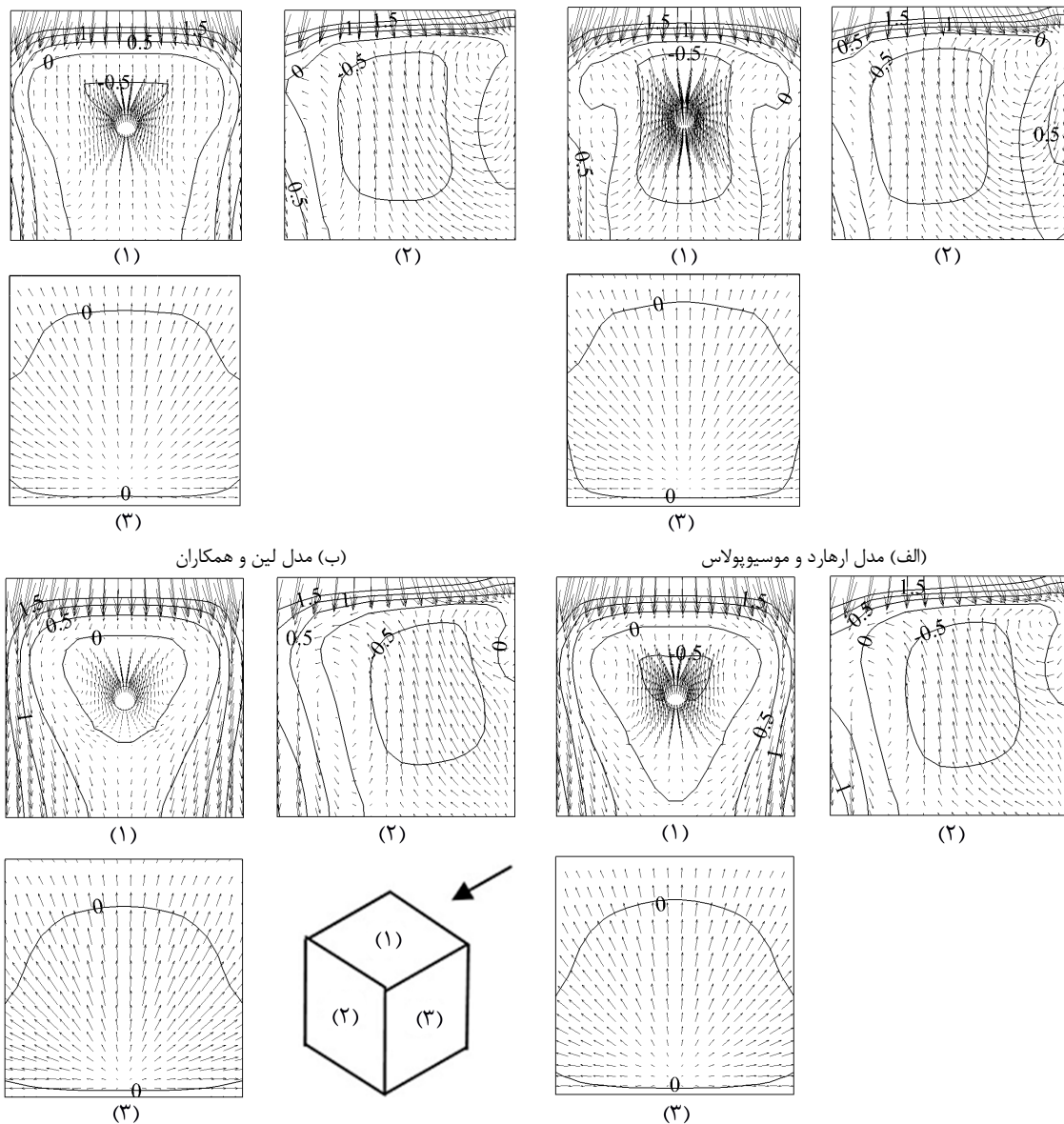
شکل ۳ بردارهای سرعت و کانتورهای مولفه در راستای جریان متوسط u بر روی (۱) سقف، (۲) دیوار بادپناه و (۳) دیوار جانبی ساختمان مدل
