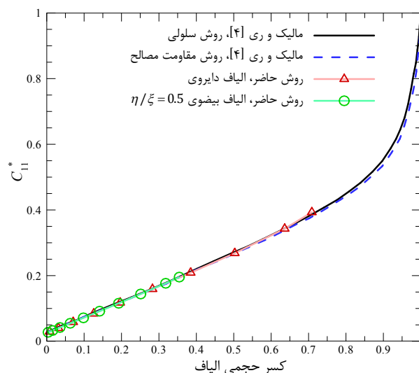
شکل ۷ تغییرات ضریب الاستیک نرمالیزه شده C_{11}^* کامپوزیت پیزوالکتریکی الیافی نسبت به کسر حجمی الیاف در حالت پولاریزاسیون عرضی
