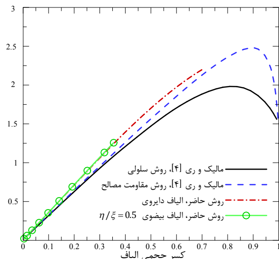
شکل ۶ تغییرات ضریب دی‌الکتریکی نرمالیزه شده \kappa_{33}^* کامپوزیت پیزوالکتریکی الیافی نسبت به کسر حجمی الیاف در حالت پولاریزاسیون عرضی
