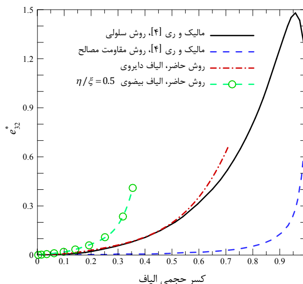
شکل ۴ تغییرات ضریب پیزوالکتریکی نرمالیزه شده e_{32}^* کامپوزیت پیزوالکتریکی الیافی نسبت به کسر حجمی الیاف در حالت پولاریزاسیون عرضی
