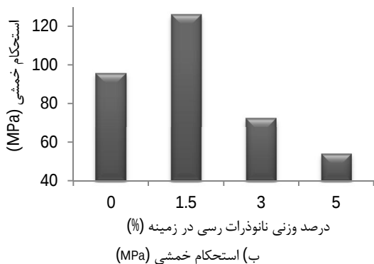
شکل 6 تغییرات خواص خمشی نمونه‌های نانوکامپوزیتی سخت شده با هاردنر تتا
