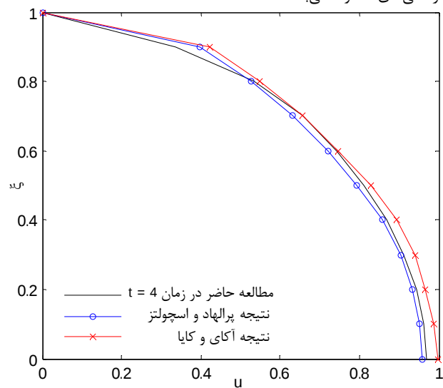
شکل 2 مقایسه سرعت محوری در شش حاضر با نتایج [23] و [25]
