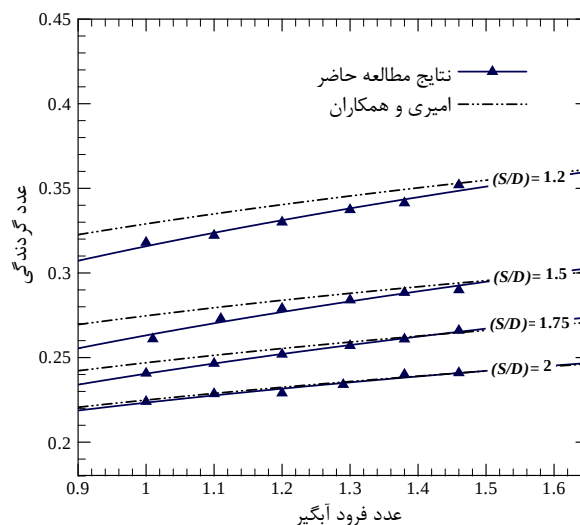
شکل 5 تغییرات عدد گردندگی گرداب های تشکیل شده در آبگیر افقی بر حسب عدد فرود و عمق استغراق نسبی
