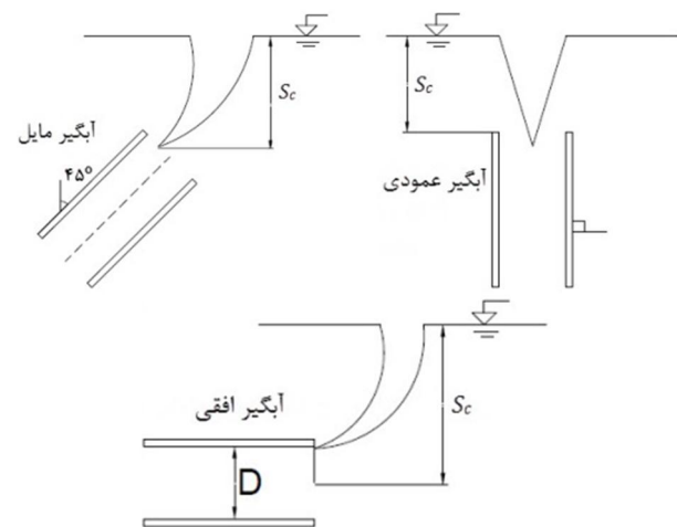
شکل 3 زوایای آبگیری مورد مطالعه
