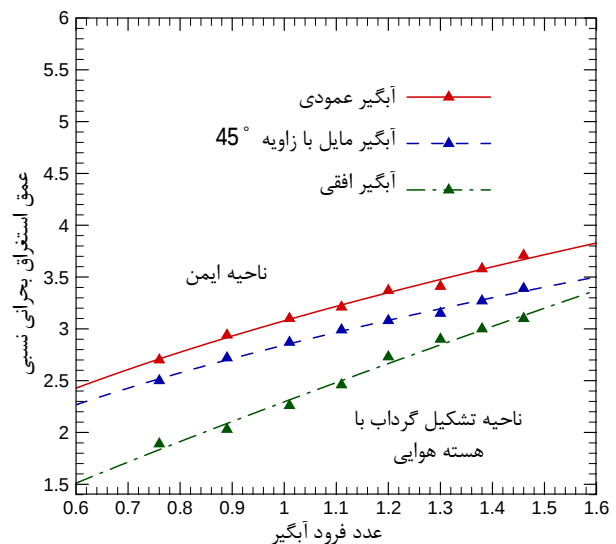
شکل 13 تغییرات عمق استغراق بحرانی نسبی برحسب عدد فرود و زاویه آبگیری
