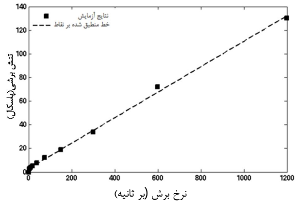
شکل 6 نمودار تنش برشی سیال مگنتورئولوژیکال بر حسب نرخ برش
