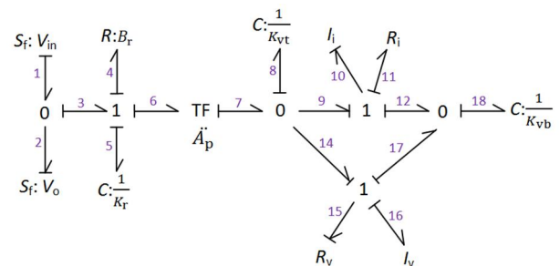
شکل 4 مدل باند گراف دسته موتور مگنتورئولوژیکال
