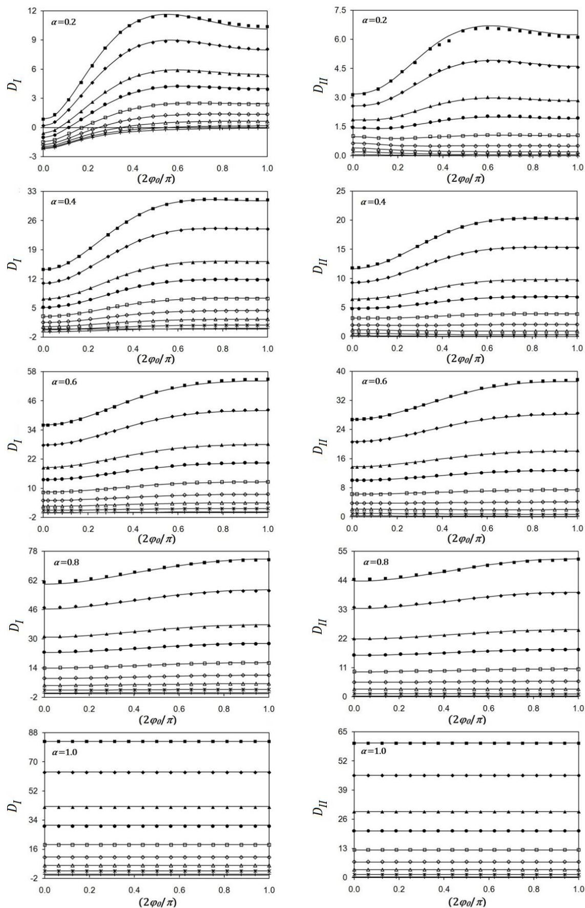
شکل ۵ ضرایب توابع وزن مود ترکیبی ترک زیرسطحی بیضوی برای \alpha ها، \beta ها و \eta_0 های مختلف
