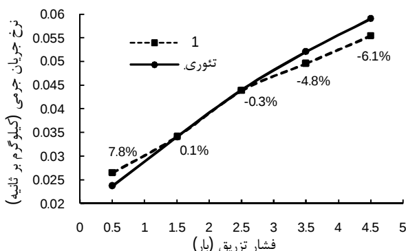
شکل 9 مقایسه منحنی تئوری دبی جرمی بر حسب فشار با افشانک شماره 1-درصد خطای میانگین نسبت به پیش‌بینی طراحی
