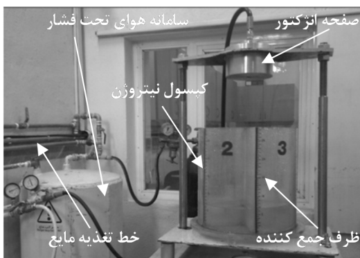
شکل 4 تصویر دستگاه آزمون پاشش (آزمایشگاه پیشران‌ش تربیت مدرس)
