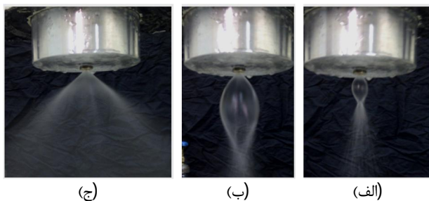
شکل 7 تصویری از پاشش سیال- از الف تا ج فشار افزایش داده شده است
